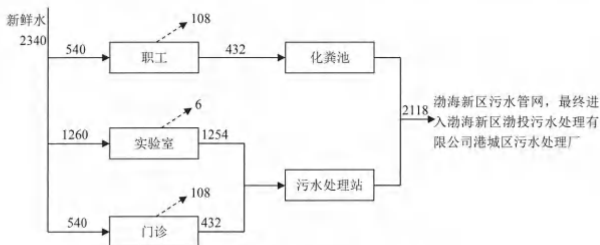
图 3-1 项目水平衡图 单位：m 3 /a
