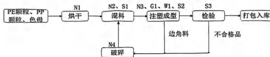
料盘生产工艺流程图
